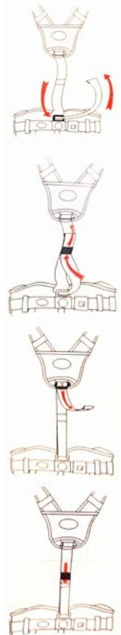
Fig. 10 Harrier Chest (+) kobles sammen med sitteselen på ryggen. Stropen på brystselen treies gjennom spennen på sitteselen, gjennom strikken og opp gjennom spennen på brystselen. Stram etter behov og pakk bort overskytende bånd under strikken.
