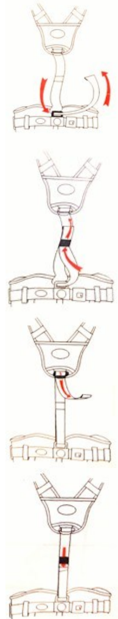
Fig. 10 Harrier Chest (+) kobles sammen med sitteselen på ryggen. Stropen på brystsele trees gjennom spennen på sitteselen, gjennom strikken og opp gjennom spennen på brystsele. Stram etter behov og pakk bort overskytende bånd under strikken.
